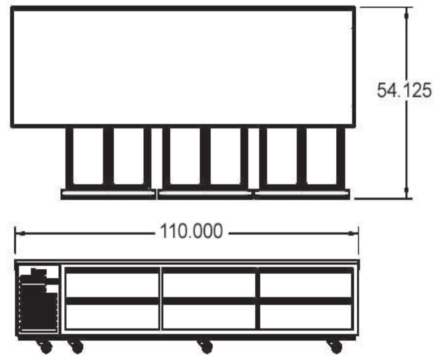
Elevation - TE110HT
