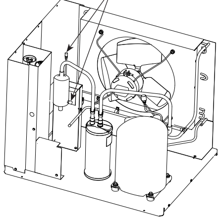
التوصيلات البديلة لصمامات شريدن بوحددة التكتيف
