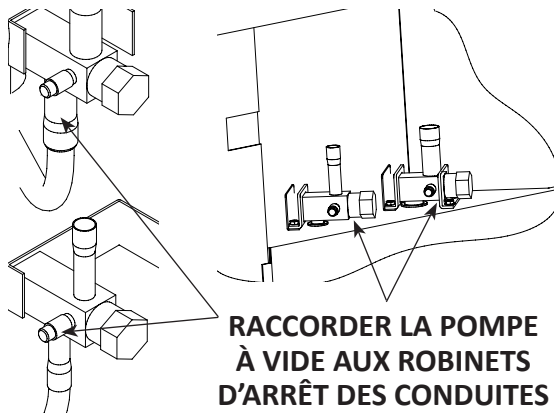
EMPLACEMENT DES RACCORDEMENTS DE CONDUITE
