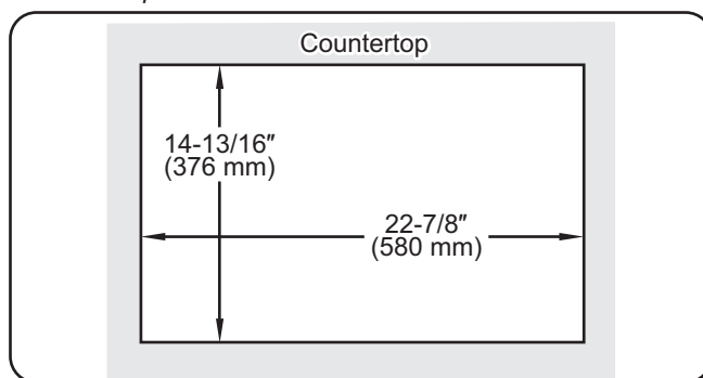
Découpe du plan de travail
