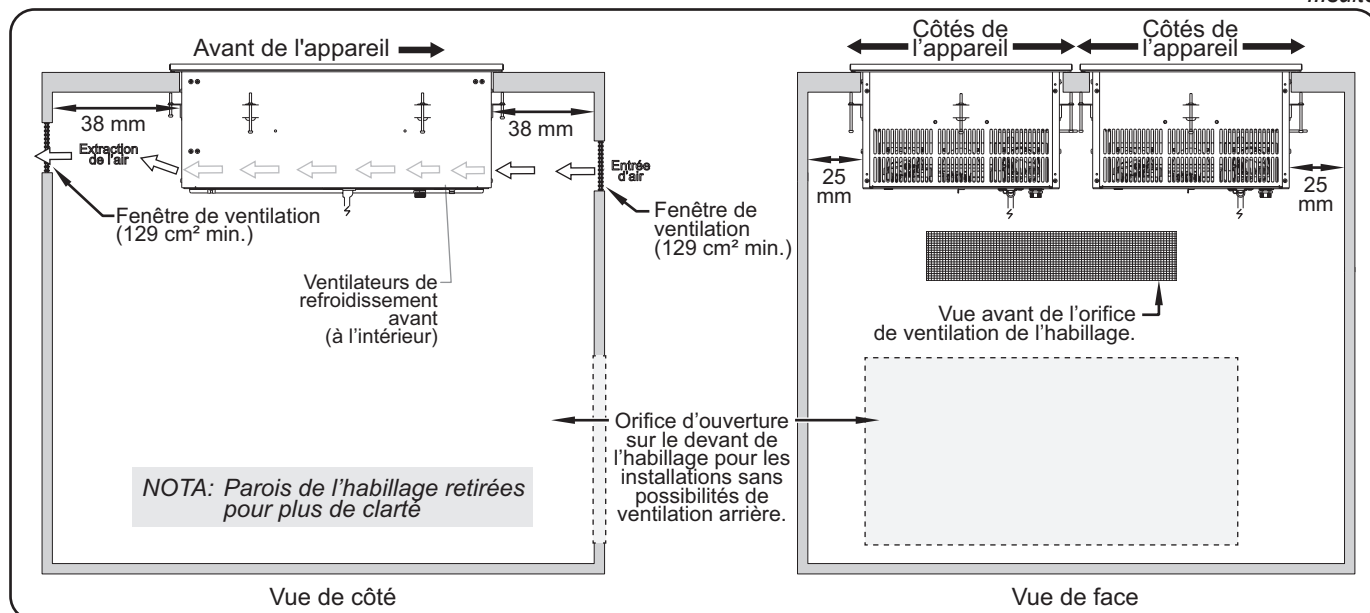
Distances minimales de montage
