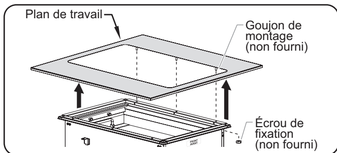
Fixation des goujons de montage
