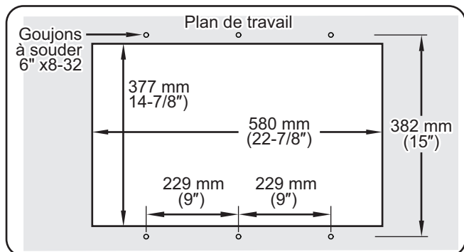
Dimensions pour l'installation avec des goujons de montage
