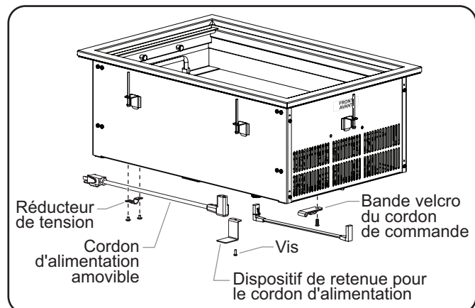
Installation du cordon d'alimentation amovible et du dispositif de retenue.
