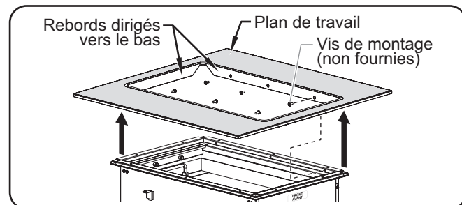
Installation sous plan à rebords
